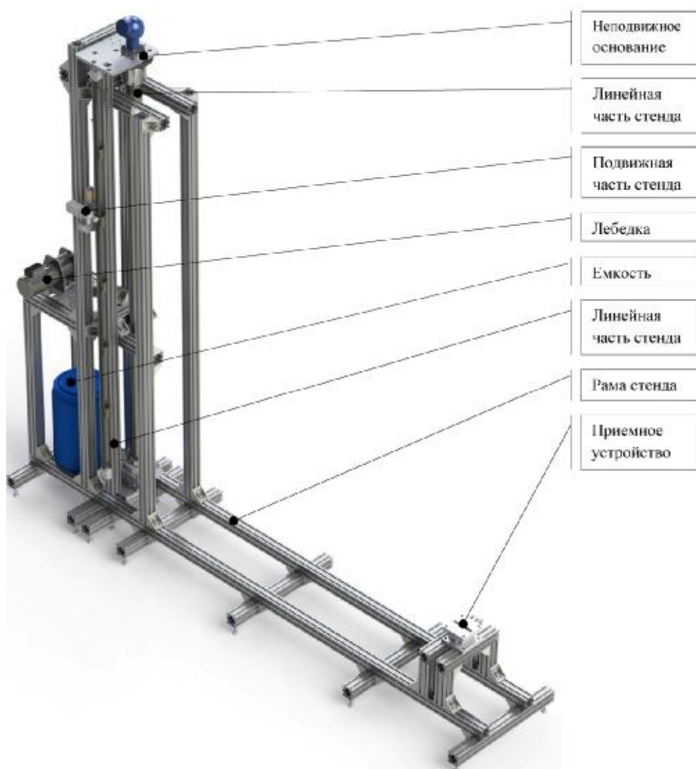
Рисунок 3. Стенд с непосредственным изменением уровня
