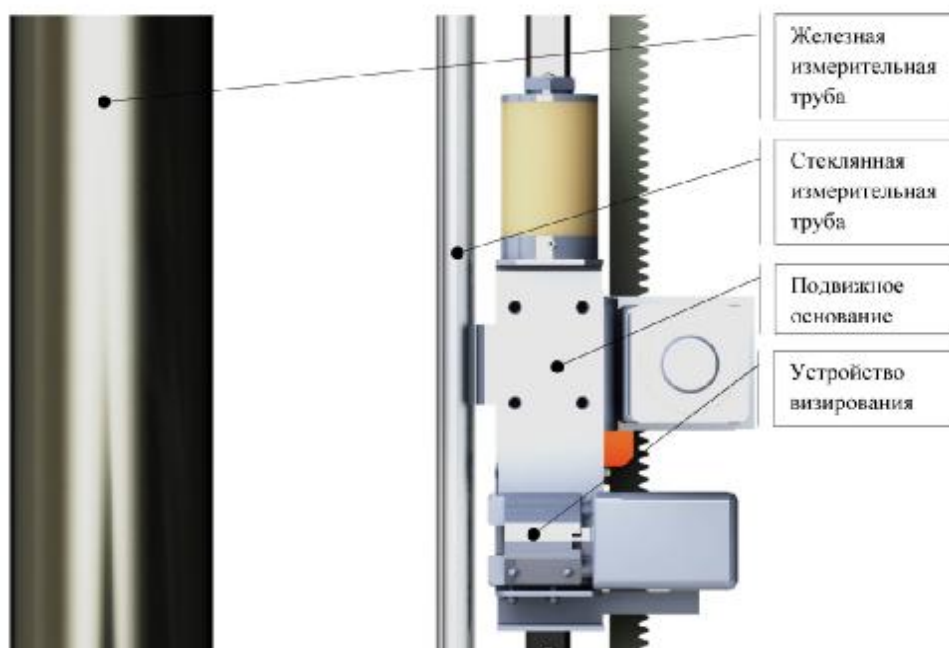
Рисунок 4. Подвижное основание стенда с непосредственным изменением уровня
