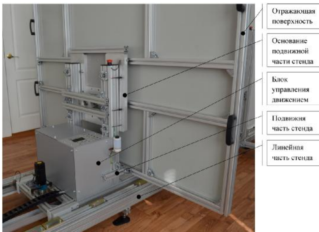
Рисунок 1. Линейная и подвижная части стенда
