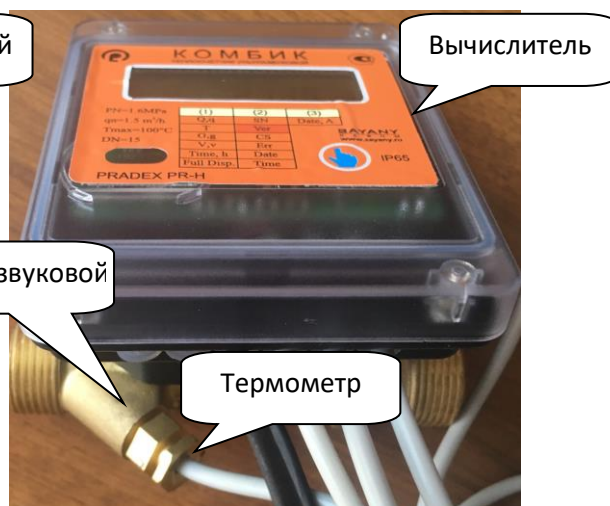
Рисунок 2 - Теплосчетчик «Комбик U» (ультразвуковой ПР)
