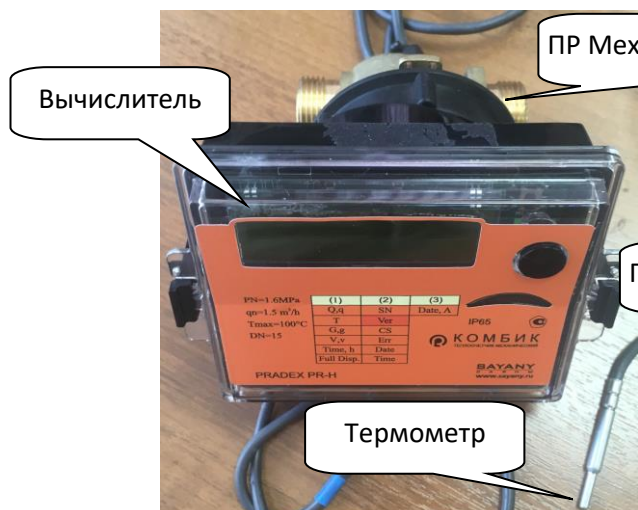
Рисунок 1 - Теплосчетчик «Комбик М» (механический ПР)
