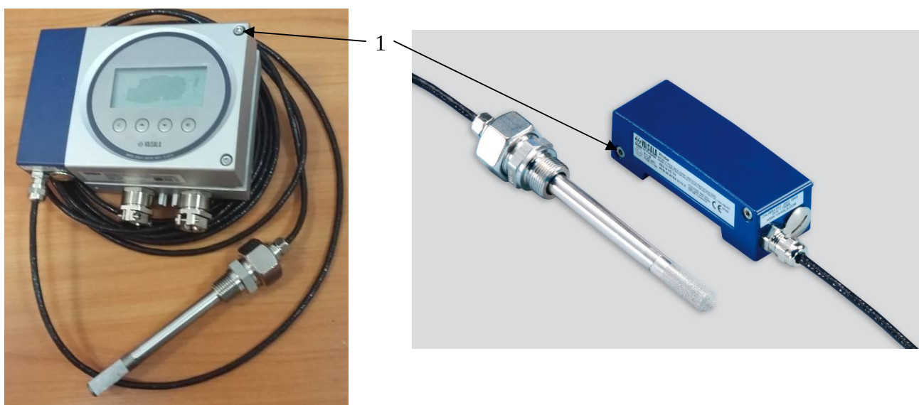
Рисунок 1 - Общий вид термогигрометра НМТ360. 1 - пломба после монтажа
