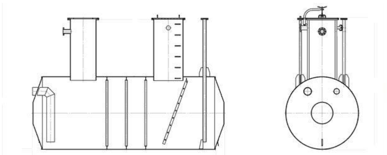
Рисунок 1 - Эскиз РГС-12,5
