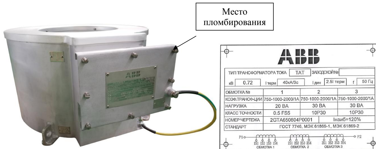
Рисунок 1 – Общий вид и место пломбирования трансформаторов тока встроенных ТАТ; вид таблички технических данных трансформаторов
