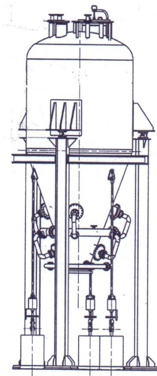
Рисунок 1 - Чертеж весов
