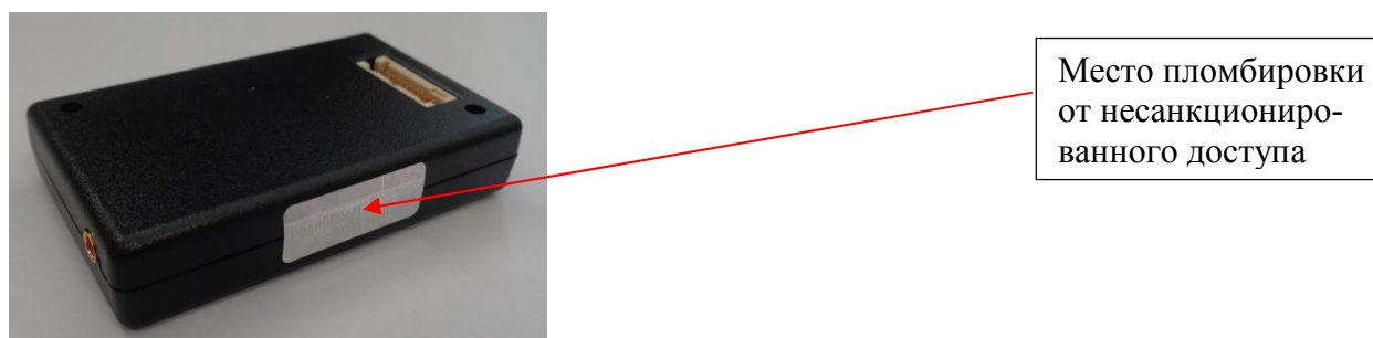
Рисунок 3 - Место пломбировки от несанкционированного доступа (вариант пломбировки № 2)
