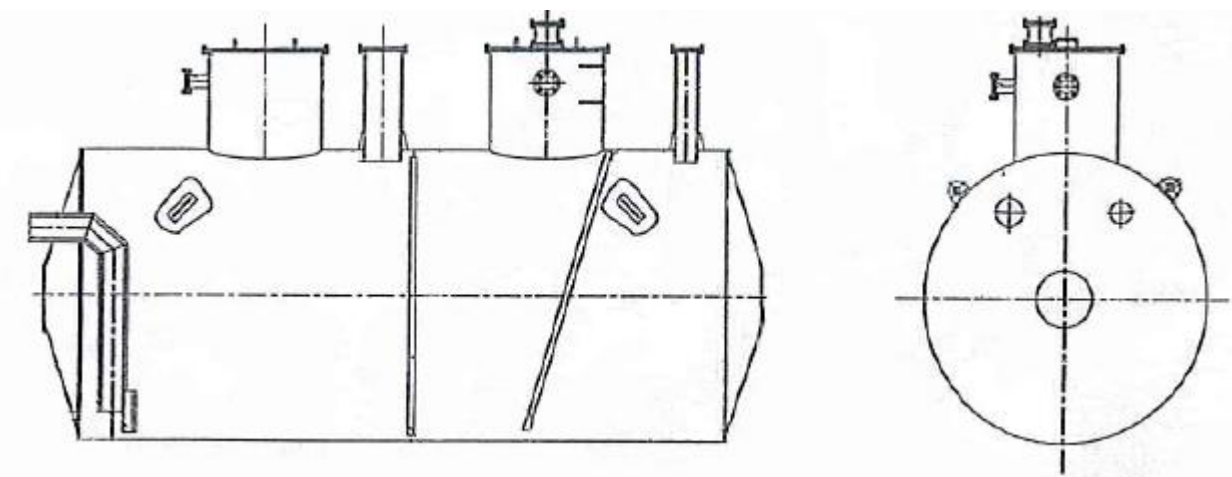
Рисунок 1 - Общий вид эскиза резервуара РГС-20
