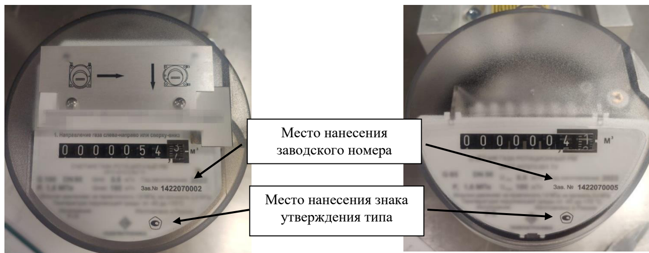
Рисунок 2 – Место нанесения заводского номера, знака утверждения типа
