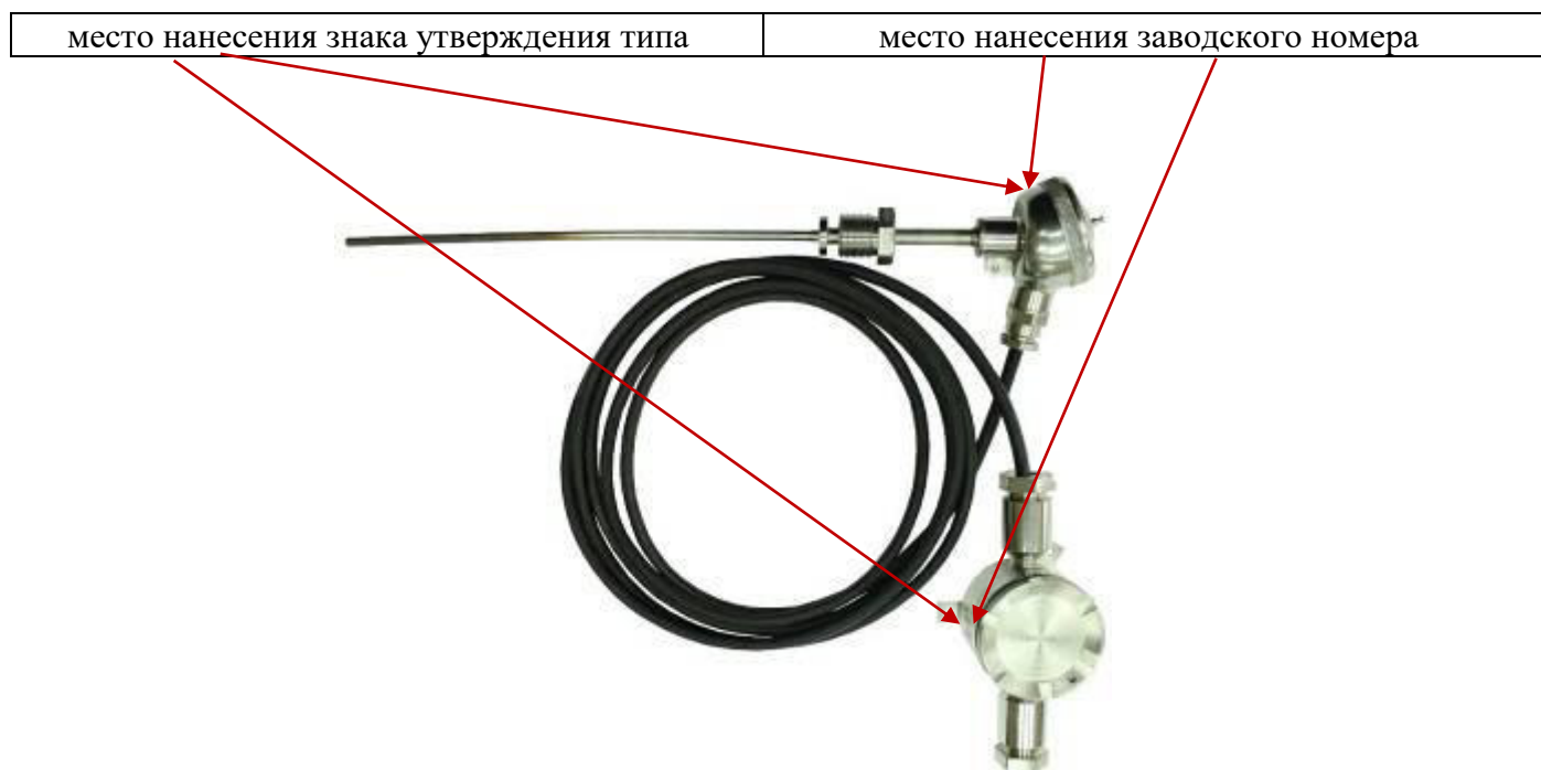
Рисунок 12 - Общий вид ТП с выносным ВП
