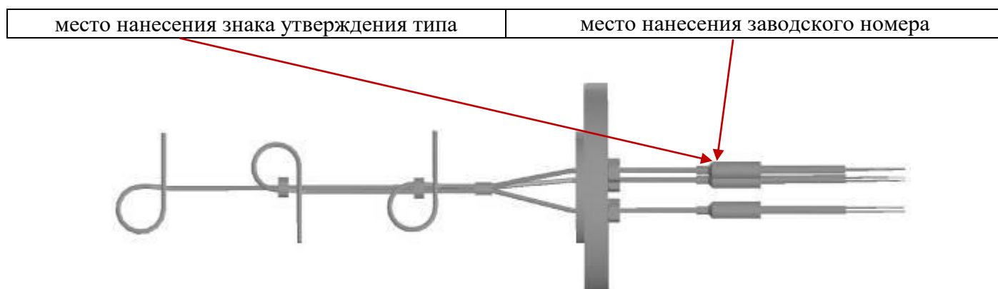
Рисунок 10 - Общий вид ТП модификаций ТХА/1-2988, ТХК/1-2988, ТНН/1-2988, ТЖК/1-2988
