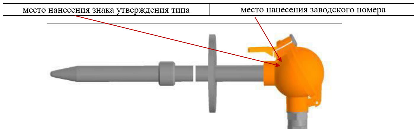
Рисунок 9 - Общий вид ТП модификаций ТХА/1-2888, ТХК/1-2888, ТНН/1-2888, ТЖК/1-2888
