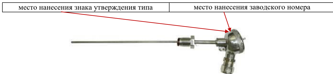
Рисунок 7 - Общий вид ТП модификаций ТХА/1-2088, ТХК/1-2088, ТНН/1-2088, ТЖК/1-2088
