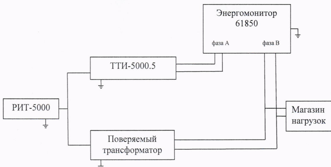
Рисунок 2 – Схема определения погрешностей коэффициента масштабного преобразования, угла фазового сдвига (для трансформаторов классов точности TPX; TPY; TPZ) и погрешности по виткам (для трансформаторов классов точности PX; PXR)
