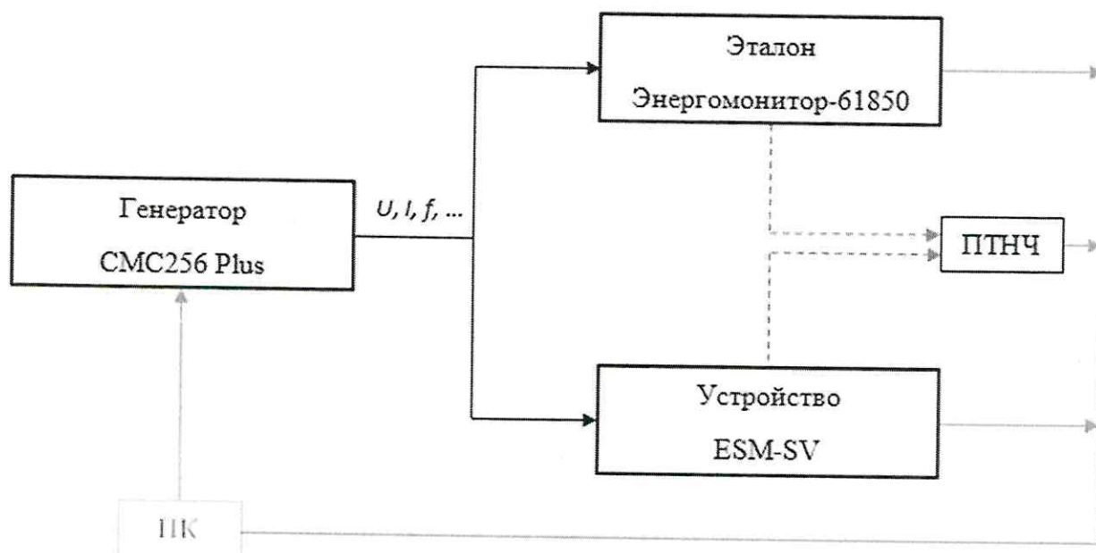
Рисунок А.2 – Схема подключения при проверке метрологических характеристик модификаций ESM-SV
