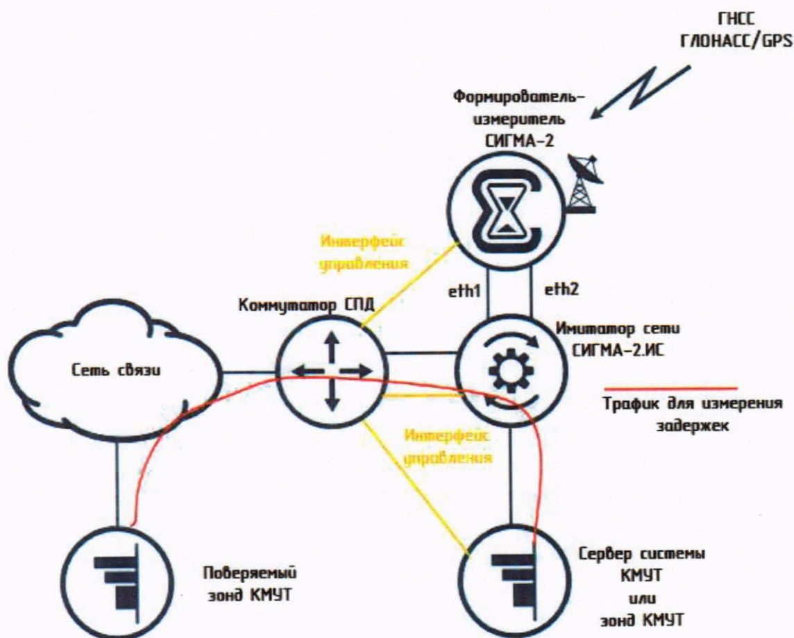
Рисунок 24 – Схема измерений для определения диапазона и погрешности измерений средней задержки передачи пакетов данных (PD)
