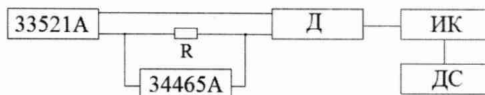
Р и с у н о к Б . 1 4 – Схема проверки канала ИК импульсного сигнала
