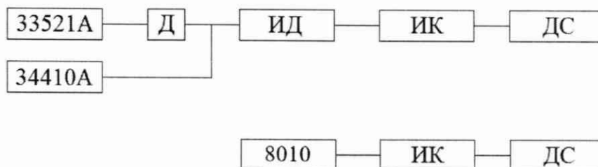
Р и с у н о к Б . 1 3 – Схема проверки ИК линейного перемещения
