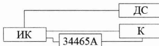
Р и с у н о к Б . 7 – Схема проверки ИК силы постоянного и переменного тока свыше 5 А
