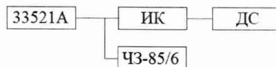
Р и с у н о к Б . 1 0 – Схема проверки ИК частоты вращения
