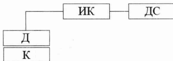
Р и с у н о к Б . 8 – Схема проверки ИК силы постоянного тока 4-20 мА
