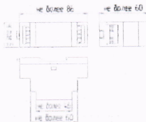
Рисунок А.5 – Преобразователь, с конструктивным исполнением Д для крепления на DIN-рейку с цифровым протоколом, или без цифрового протокола. Степень защиты оболочки IP20
