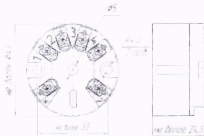
Рисунок А.3 – Преобразователь, с конструктивным исполнением Кп с цифровым протоколом или без цифрового протокола, для крепления в клеммной голове ПП. Степень защиты оболочки IP20.
