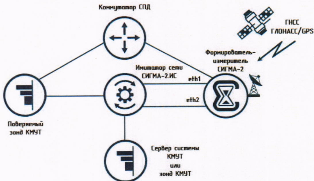
Рисунок 20 – Схема измерений для определения диапазона и погрешности измерений средней задержки передачи пакетов данных (PD)
