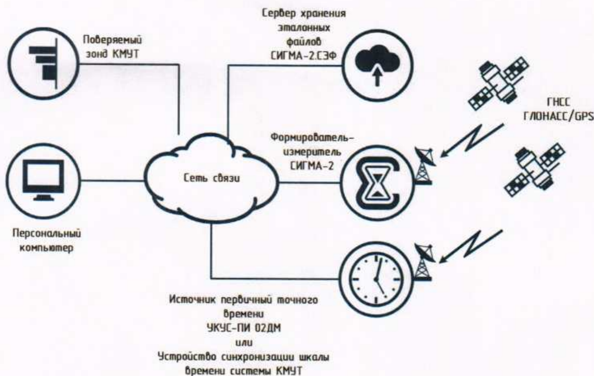
Рисунок 5 – Схема измерений при поверке зонда КМУТ, установленного на сети связи
