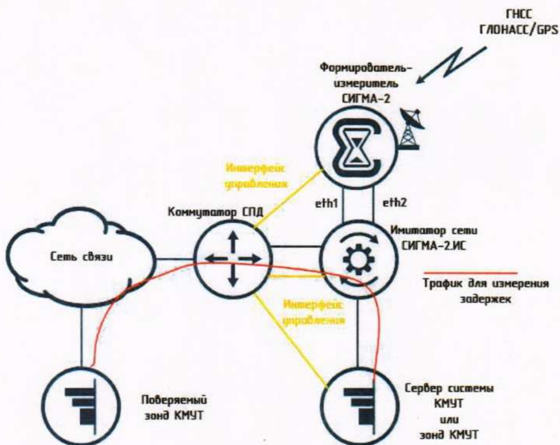
Рисунок 24 – Схема измерений для определения диапазона и погрешности измерений средней задержки передачи пакетов данных (PD)
