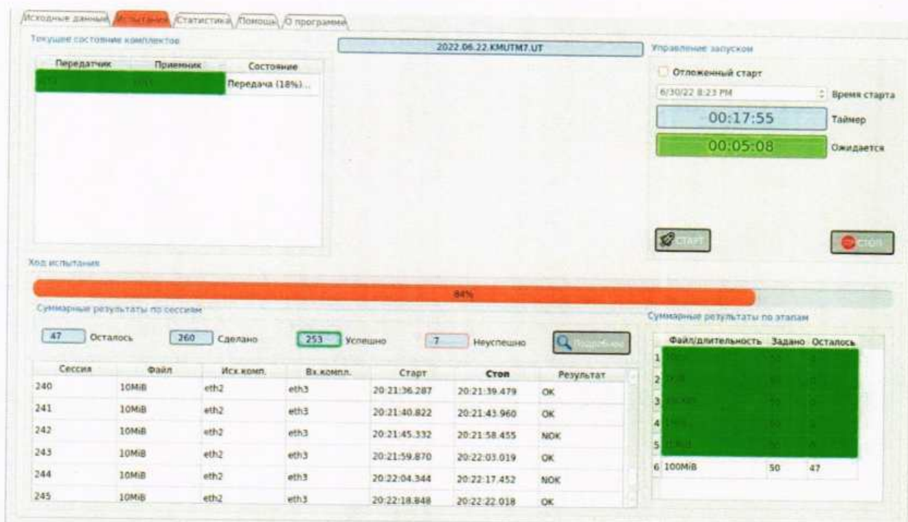
Рисунок 11 – Промежуточное индицирование результата испытаний (режим «Информация»)
