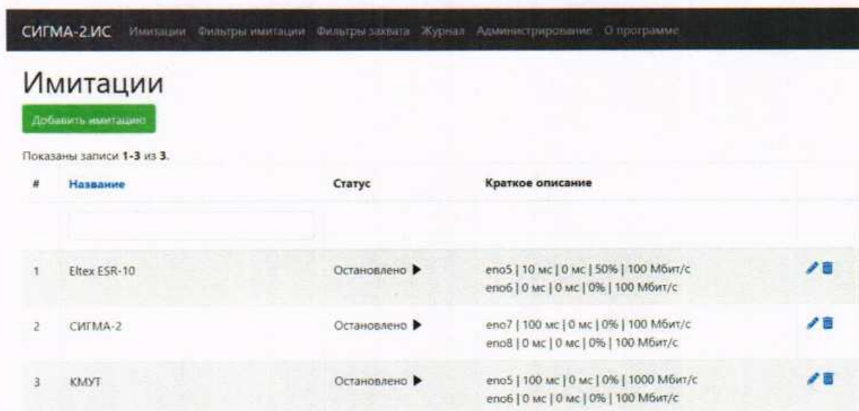
Рисунок 22 – Страница управления имитациями прибора СИГМА-2.ИС
