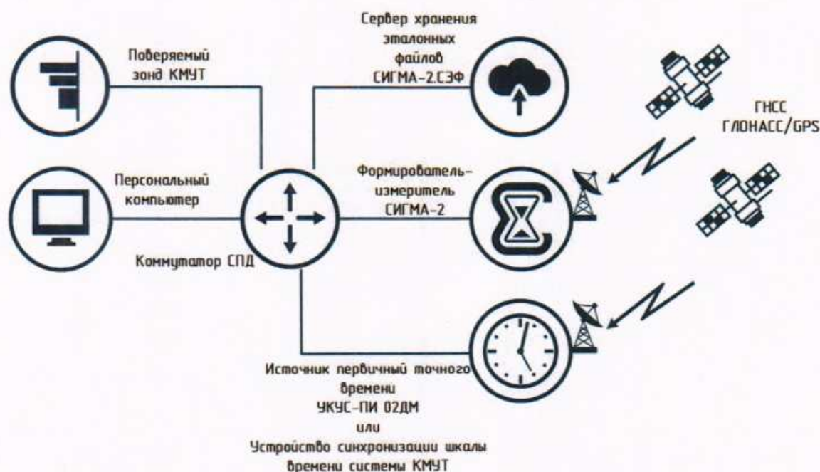
Рисунок 4 – Схема измерений при поверке зонда КМУТ
