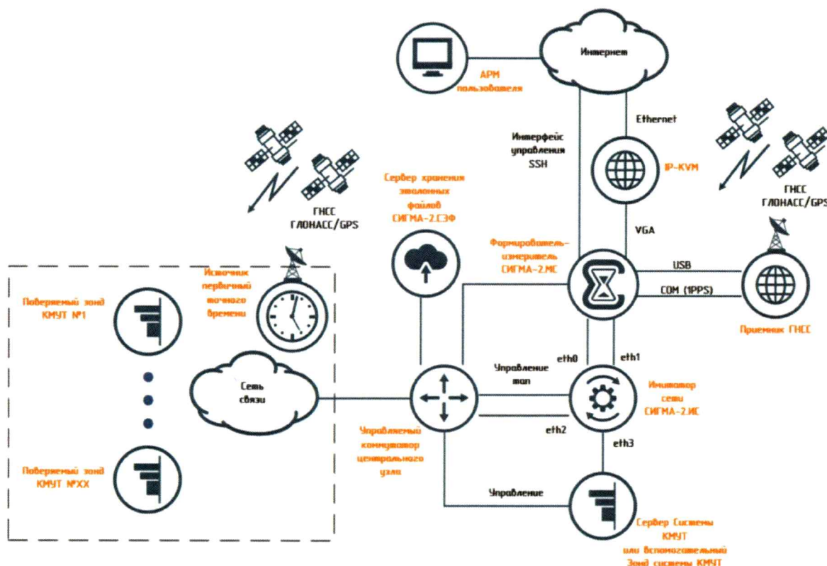
Рисунок 8 – Схема измерений при поверке зонда КМУТ, установленного на сети связи
