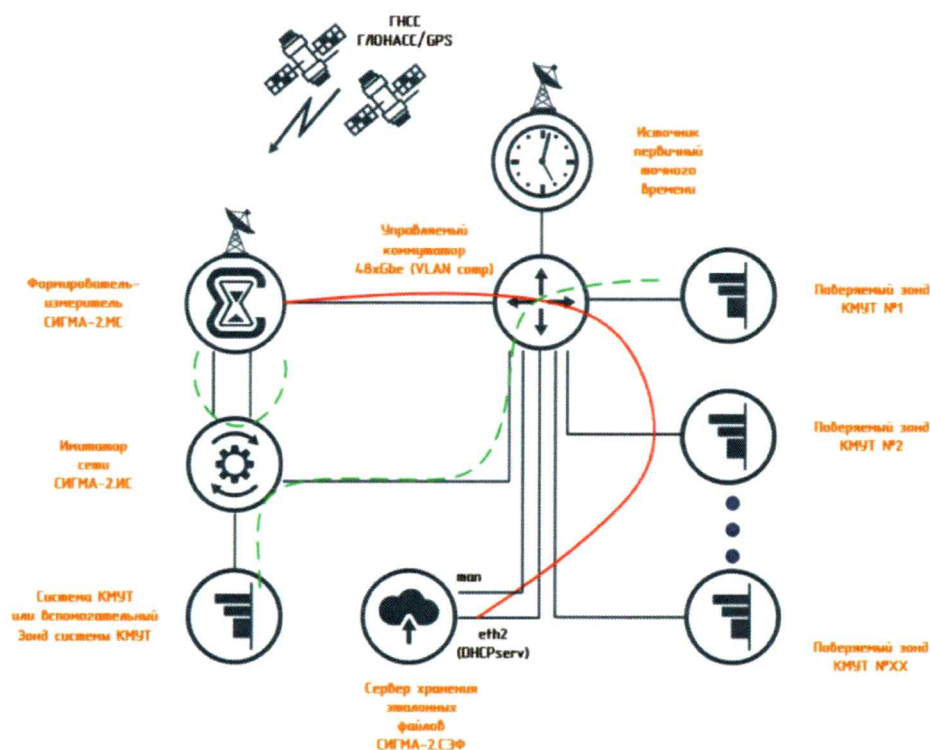
Рисунок 7 – Схема измерений при поверке зонда КМУТ
