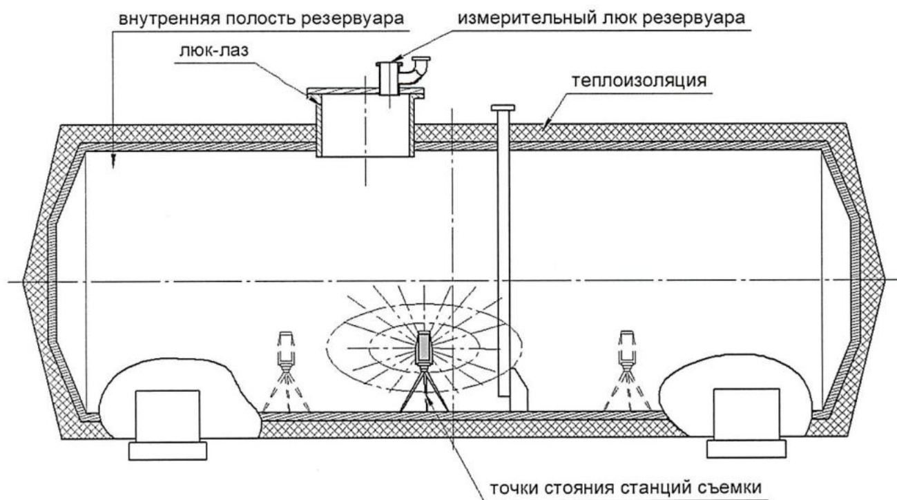
Рисунок А.3 – Схема измерений внутренней полости резервуара
