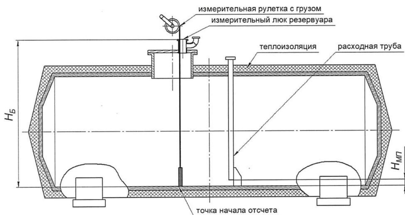
Рисунок А.2 – Схема измерений базовой высоты и измерений высоты мертвой полости
