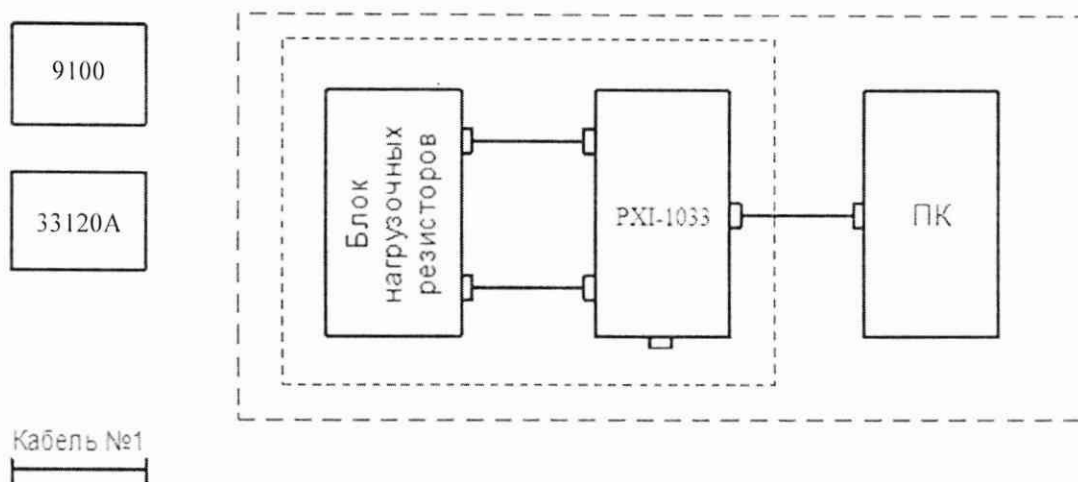
Рисунок 1 – Схема подключения комплекса для определения приведенной (к диапазону измерений) погрешности измерений электрического напряжения сигналов произвольной формы, приведенной (к диапазону измерений) погрешности измерений силы тока сигналов произвольной формы, постоянной времени при измерении электрического напряжения и силы тока сигналов произвольной формы
