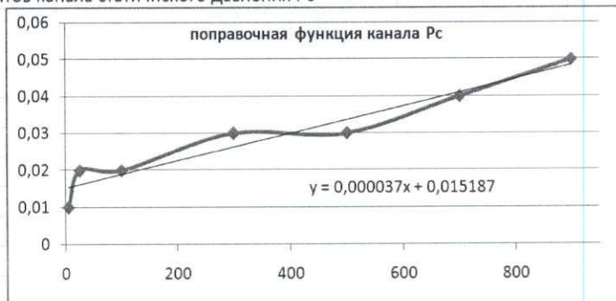
Определение поправочных коэффициентов канала статического давления P_c
