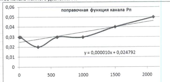
Рисунок 4 – Пример определения поправочных коэффициентов
