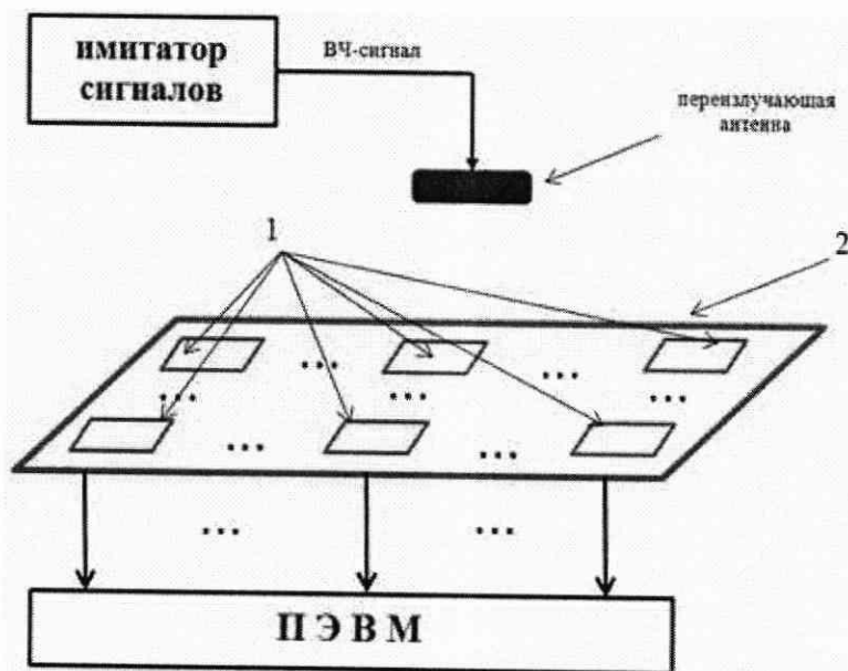
1 – устройства; 2 – СТПК ЭМБУ ЦСИ Рисунок 1 – Схема проверки работоспособности
