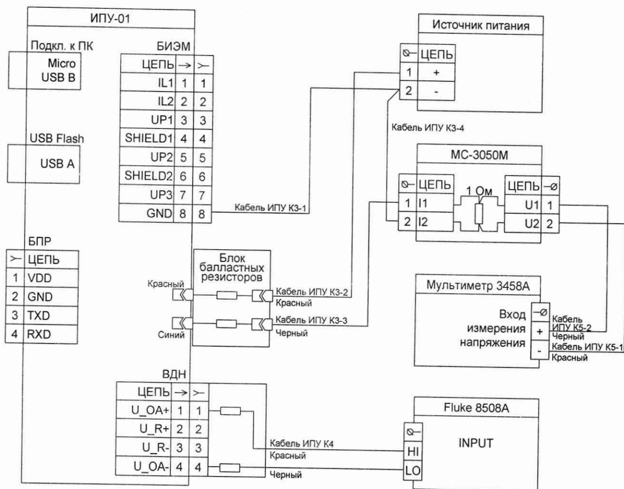
Рисунок 10.2 – Схема подключений ИПУ-01
