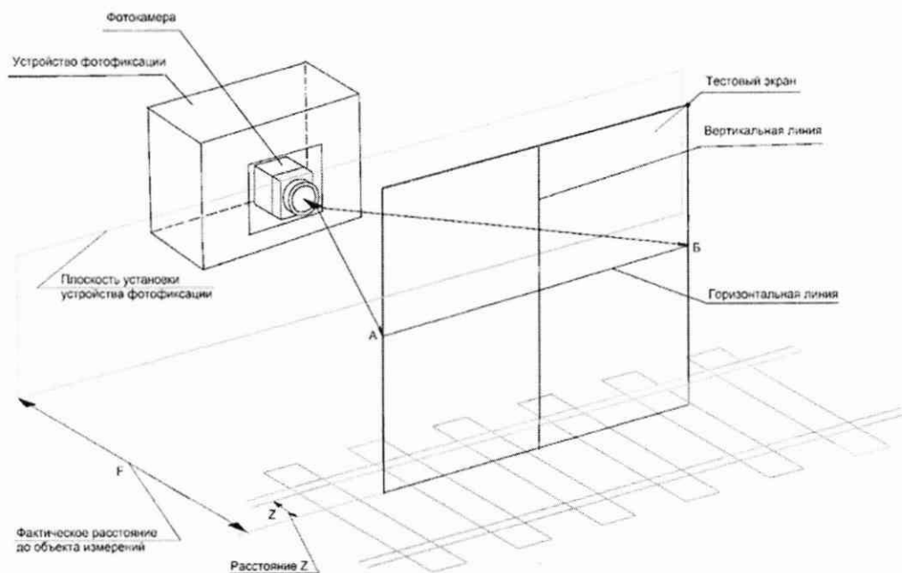
Рисунок 11- Проверка перпендикулярности положения тестового экрана.
