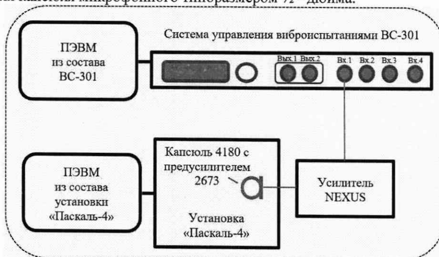
Рисунок 4 – Схема проведения измерений при определении погрешности воспроизведения рабочих частот и звукового давления в АК установки
