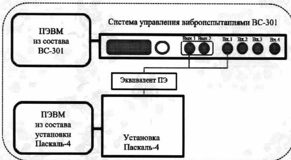
Рисунок 6 – Схема проведения измерений при определении диапазона измерений чувствительности ПЭ и относительной погрешности измерений чувствительности ПЭ по заряду
