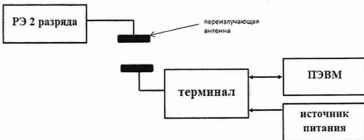
Рисунок 1 – Схема проведения измерений при проверке работоспособности, определения погрешностей измерений координат и скорости
