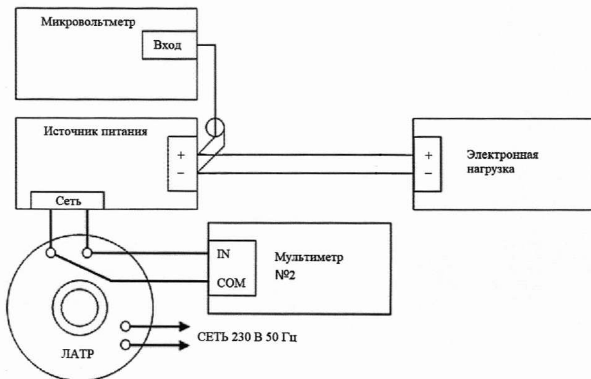
Рисунок 6 – Схема соединения № 4
