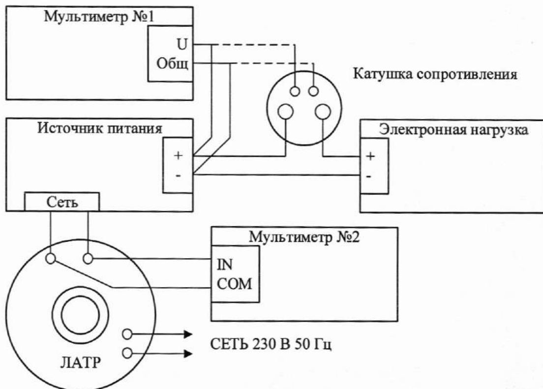
Рисунок 4 – Схема соединения № 2
