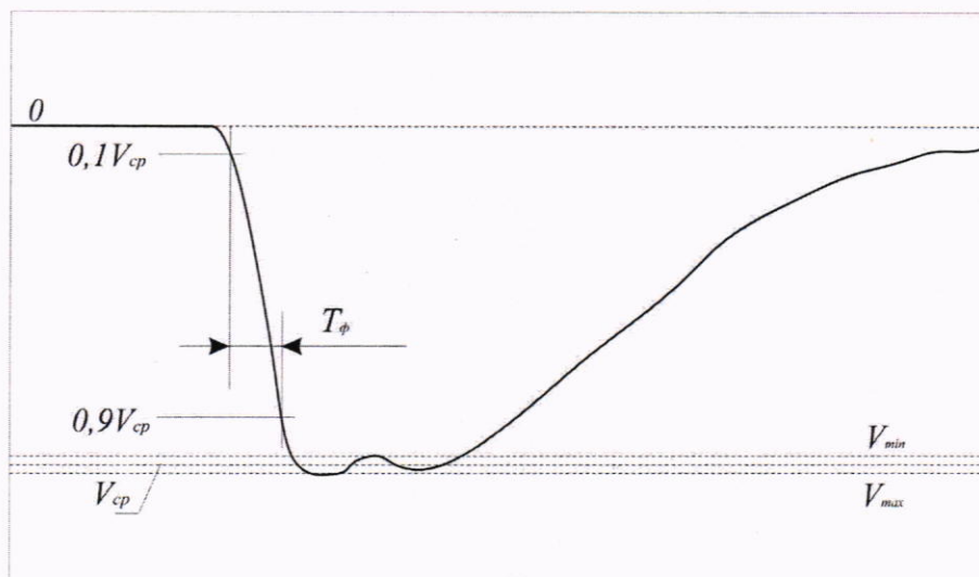
Рисунок 2 – Эпюра напряжения на выходе измерителя при определении метрологических характеристик
