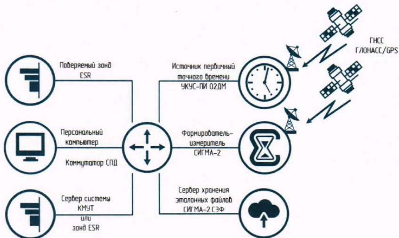
Рисунок 7 – Схема измерений при поверке зонда ESR
