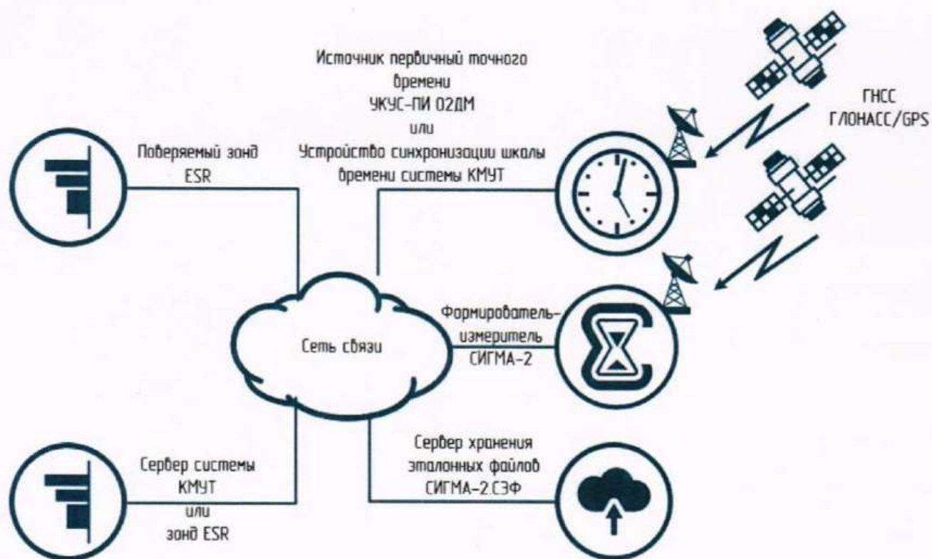
Рисунок 8 – Схема измерений при поверке зонда ESR, установленного на сети связи
