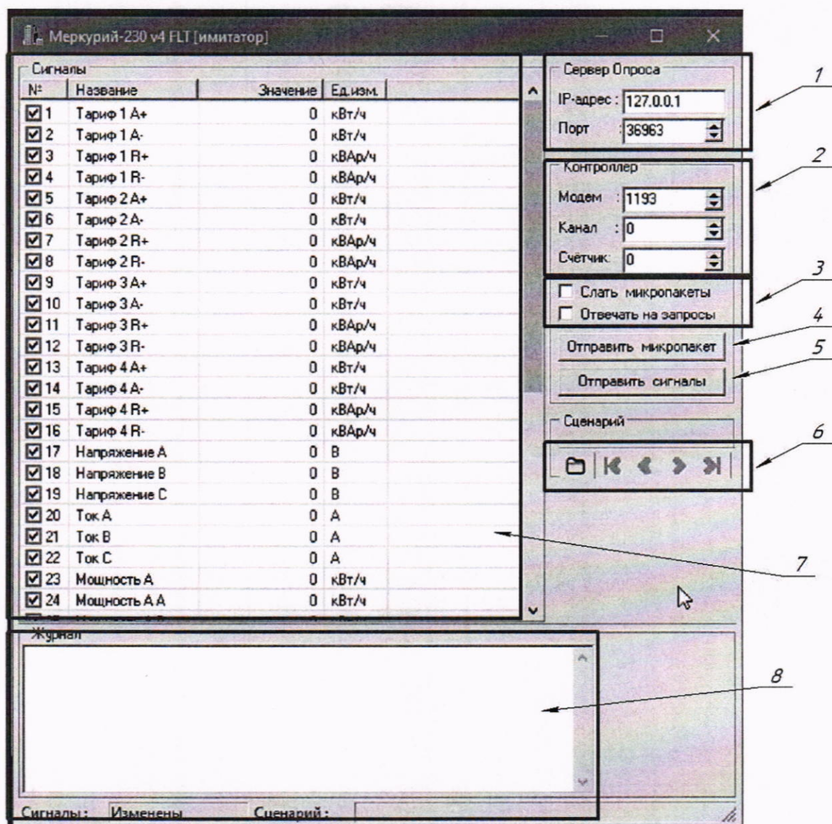
Рисунок А.13 – Элементы окна имитатора электросчетчика Меркурий-230
