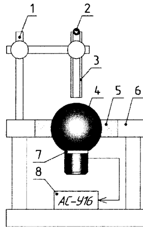
1 – кронштейн; 2 – падающий шарик; 3 – трубка направляющая; 4 – рабочее тело; 5 – прокладка виброгасящая; 6 – держатель прокладки виброгасящей; 7 – вибропреобразователь; 8 – анализатор АС-У16.
