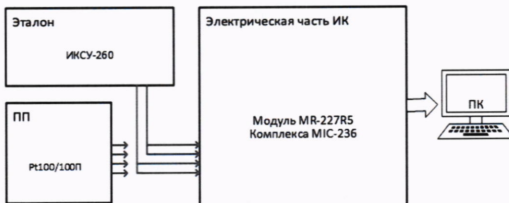
Рисунок 8 – Схема поверки ИК температур с ПИП терморезистивного типа поэлементным способом
