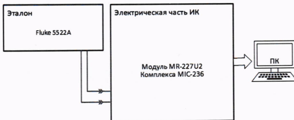
Рисунок 1 – Схема поверки ИК напряжения постоянного тока
