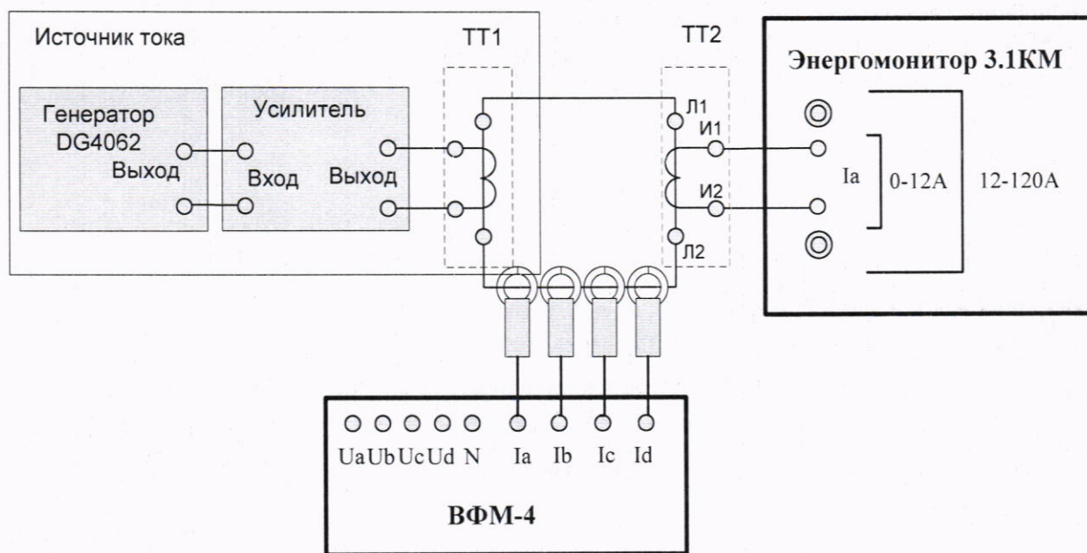
Рисунок 5 – Схема измерений для определения основной погрешности измерения тока в диапазоне выше 120 А
