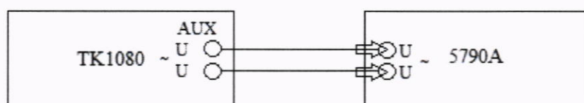
Рисунок 7 – Схема подключения калибратора к выходу AUX в режиме воспроизведения переменного электрического напряжения
