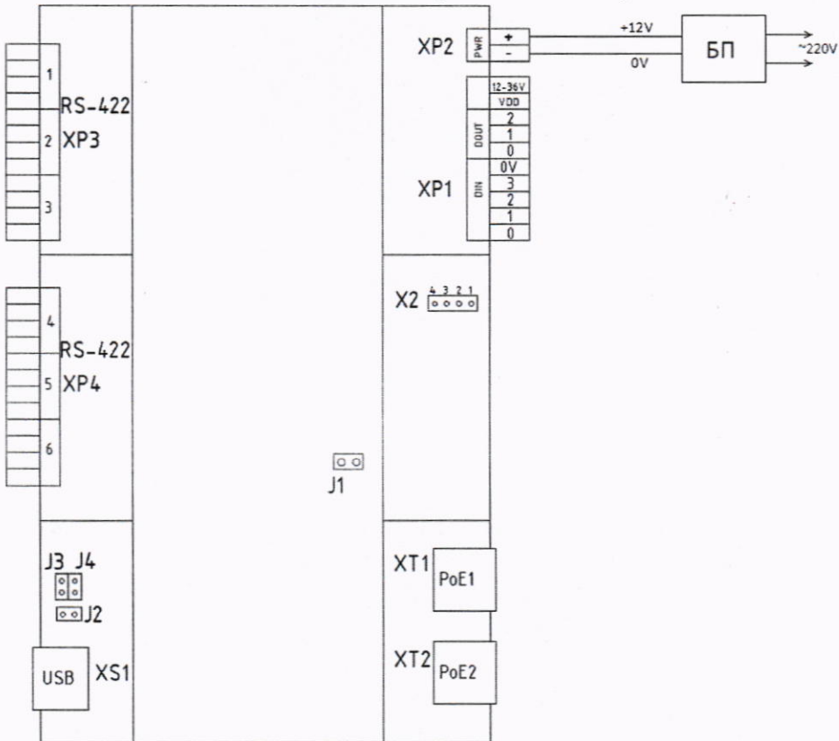
Рисунок А.1 - Схема подключения питания к УСПД
