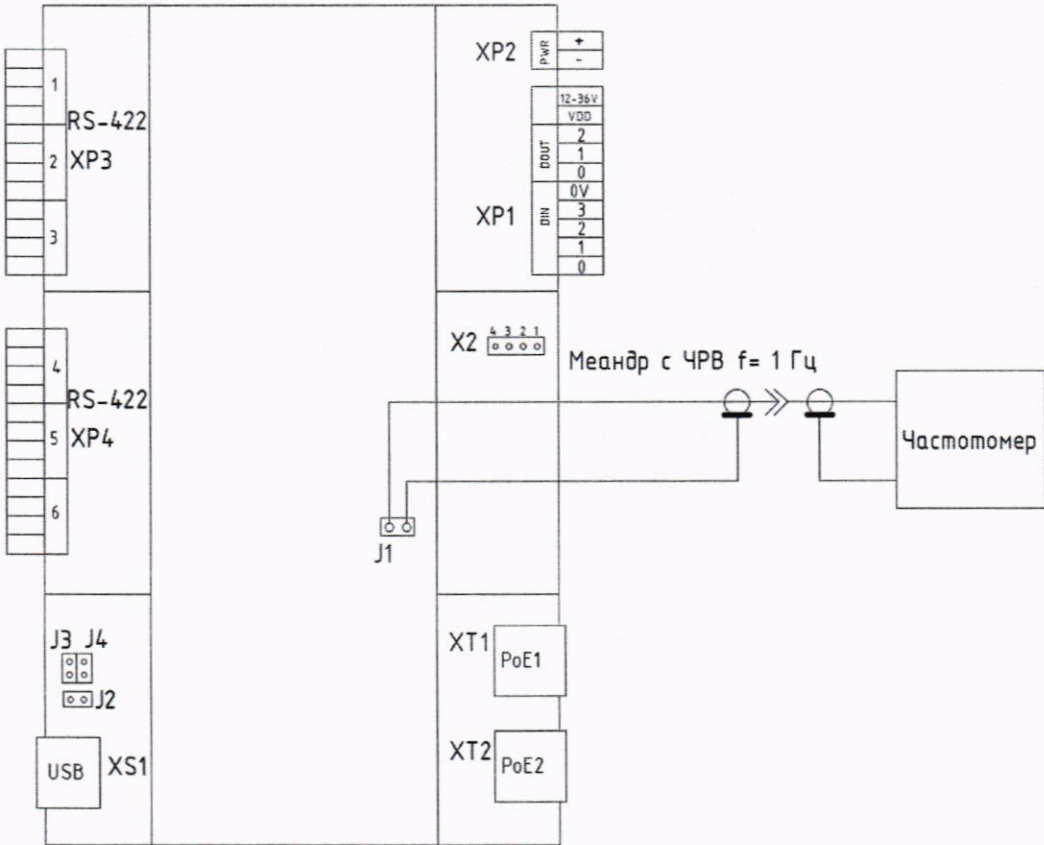
Рисунок А.2 - Схема подключения частотомера
