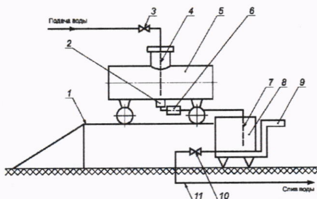
Рисунок 9.2 – Схема измерения вместимости ТМ при поверке взвешиванием вспомогательной тары при сливе поверочной жидкости из ТМ во вспомогательную тару.
