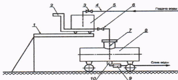
Рисунок 9.3 – Схема измерения вместимости ТМ при поверке взвешиванием вспомогательной тары при сливе поверочной жидкости из вспомогательной тары в ТМ.
