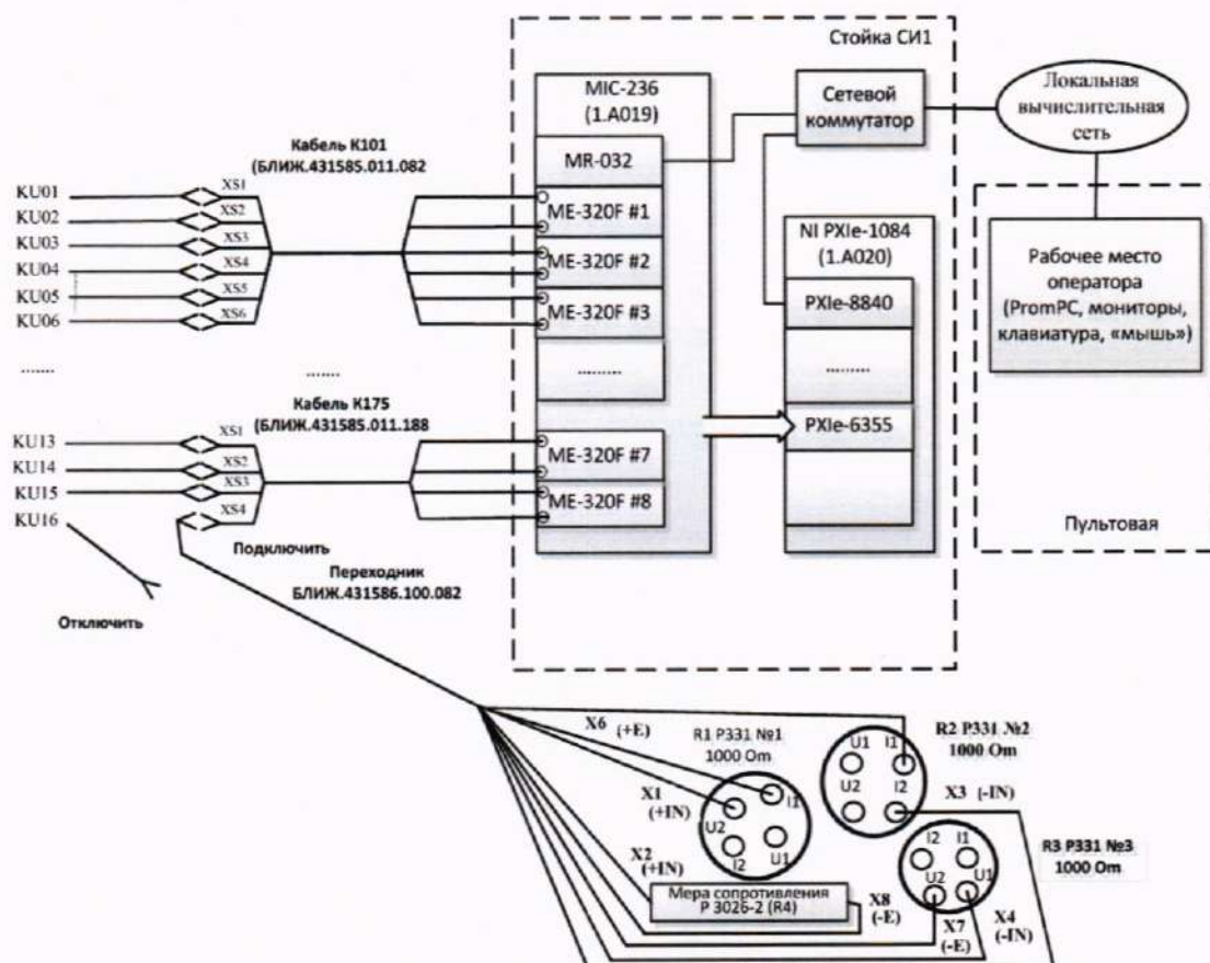
Рисунок 11 - Схема поверки электрической части ИК коэффициента преобразования напряжения постоянного тока
