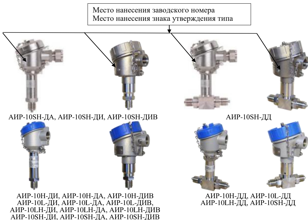
Рисунок 1 – Общий вид преобразователей давления измерительных АИР-10
