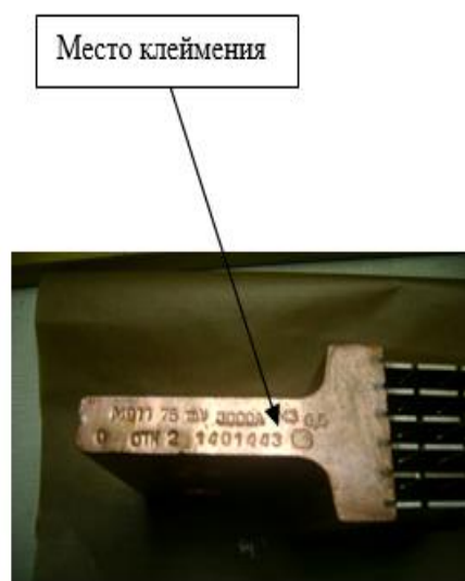
Рисунок 1 - Общий вид шунтов
