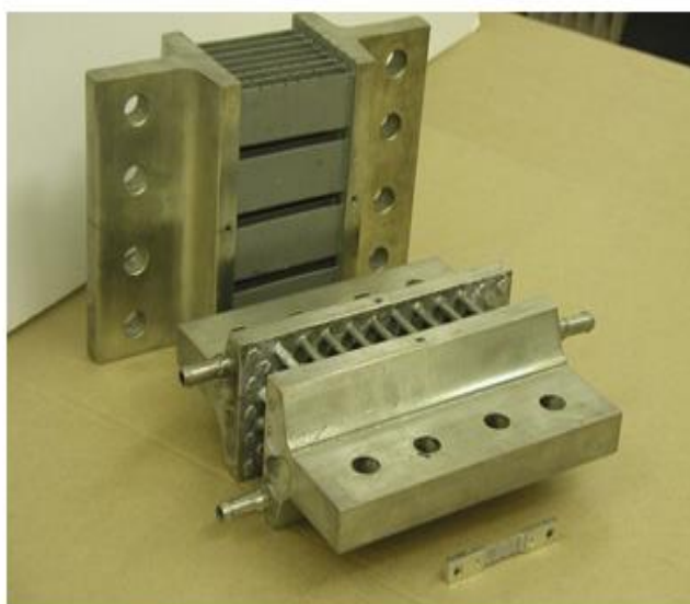
Рисунок 1 - Общий вид шунтов
