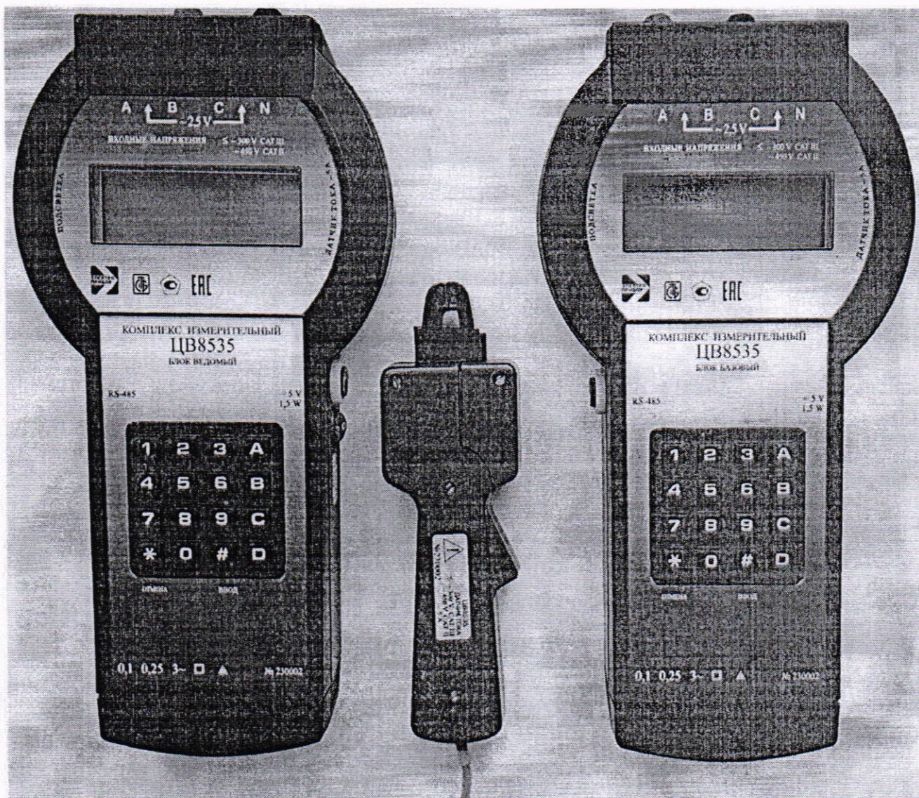
Рисунок 1.1 – Общий вид комплекса измерительного ЦВ8535
