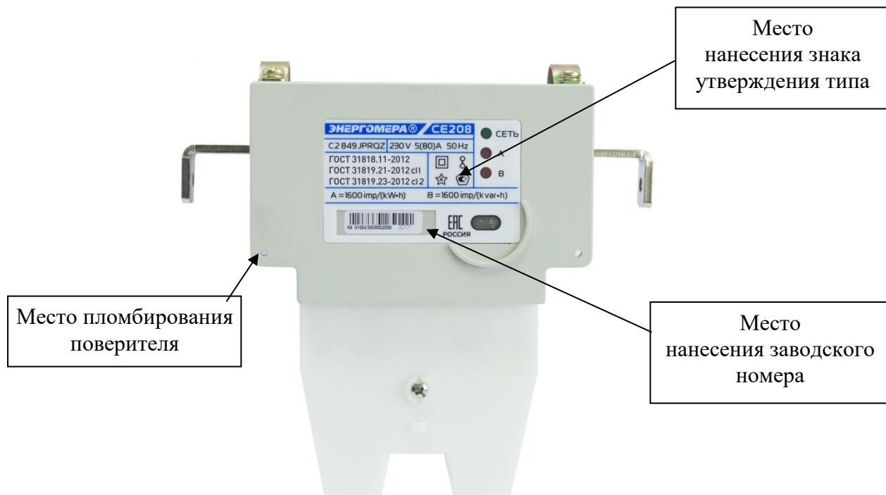
Рисунок 6 – Общий вид счетчика CE 208 C2
