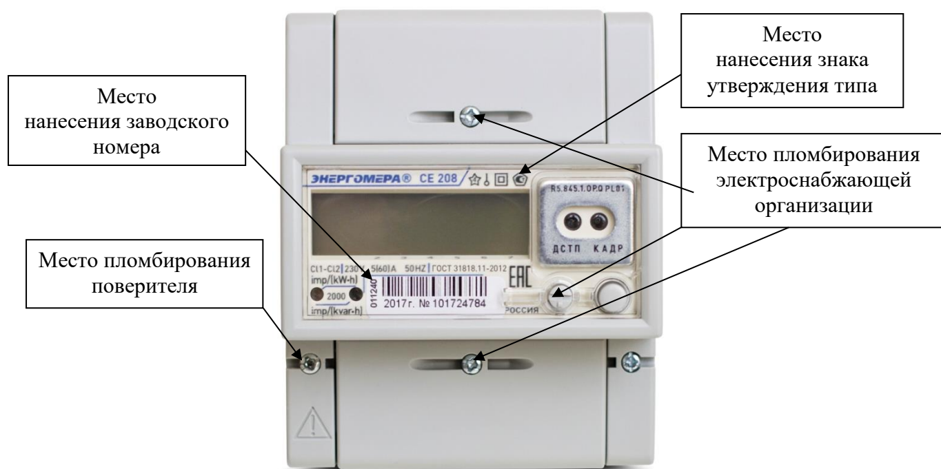
Рисунок 4 – Общий вид счетчика CE 208 R5
