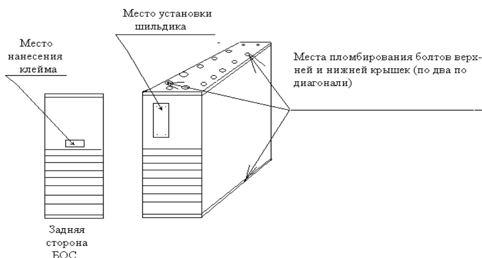
Рисунок 2 Схема пломбировки
