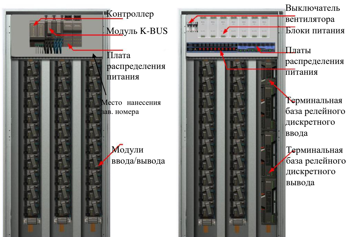
Рисунок 1 – Общий вид станции FCS
