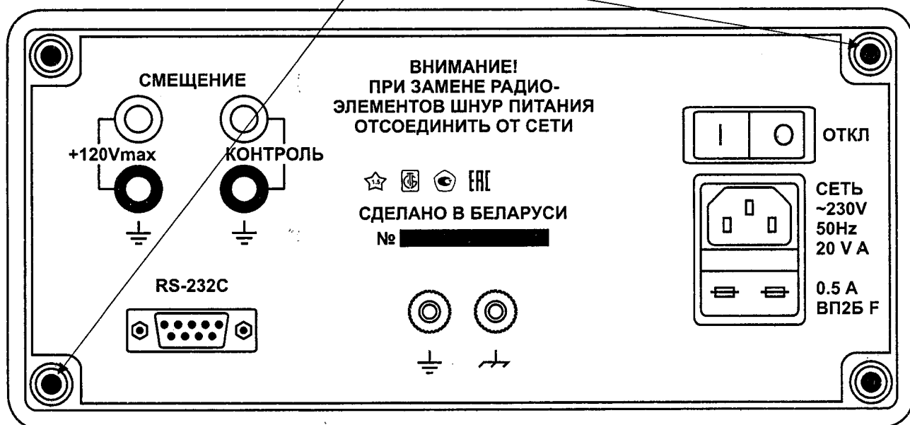
Рисунок 3.1 – Схема пломбировки от несанкционированного доступа
