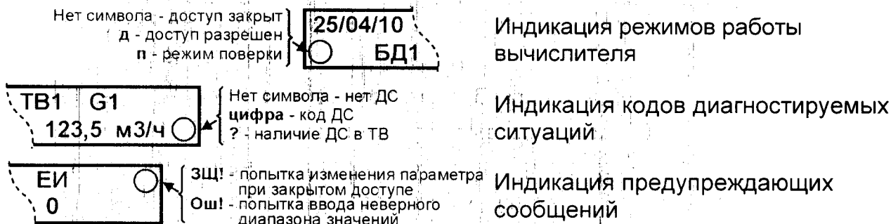
Рис. 2.2 – Индикация сервисных сообщений
