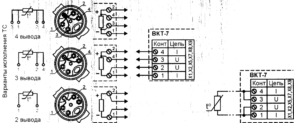
а) Подключение ТС по 4-проводной схеме б) Подключение 2-х проводных ТС Рис. 5.2 - Варианты подключения ТС
