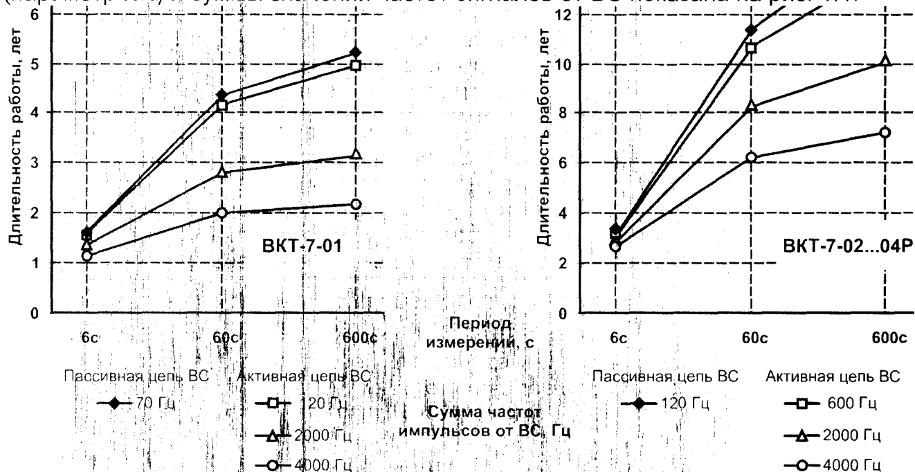
Рис. 1.1 – Зависимость ресурса батареи ВКТ-7
