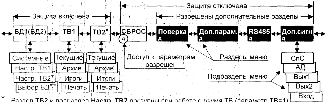
Рис. 2.5 – Структура меню вычислителя
