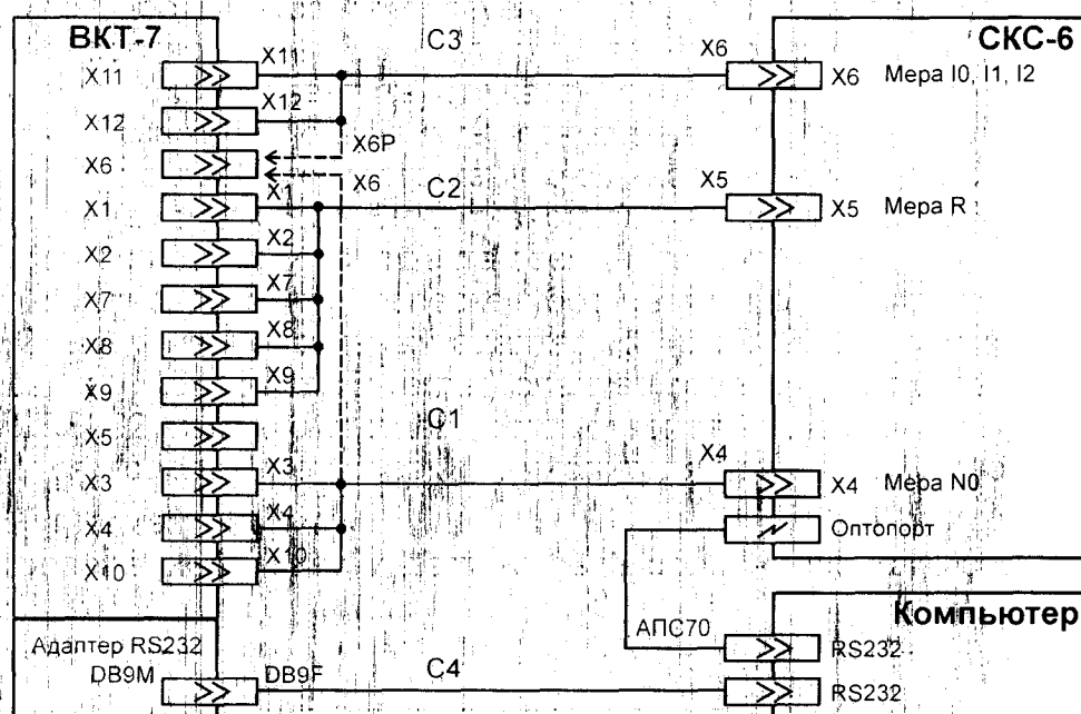
Рисунок 8.1 – Схема поверки
