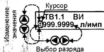
Рис. 3.2 – Пример изменения значения параметра ВИ
