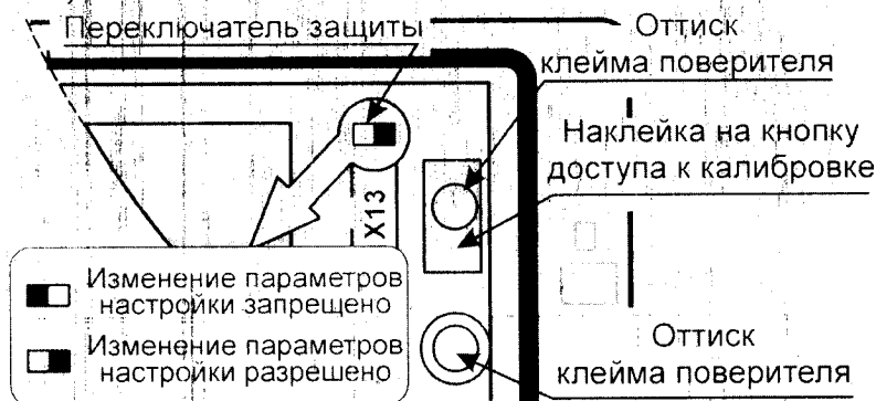
Рис. 1.2 – Места пломбирования поверителем
