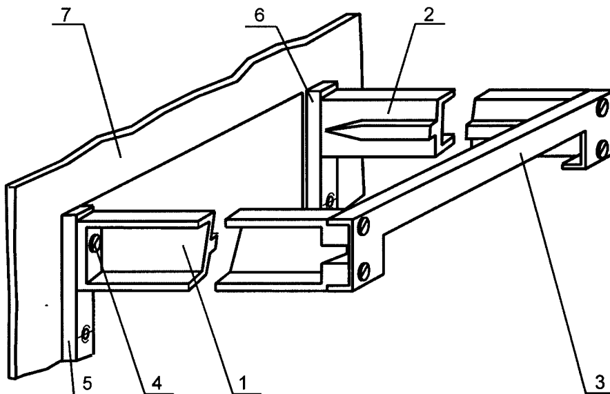
Рисунок 5 – Монтаж скобы
