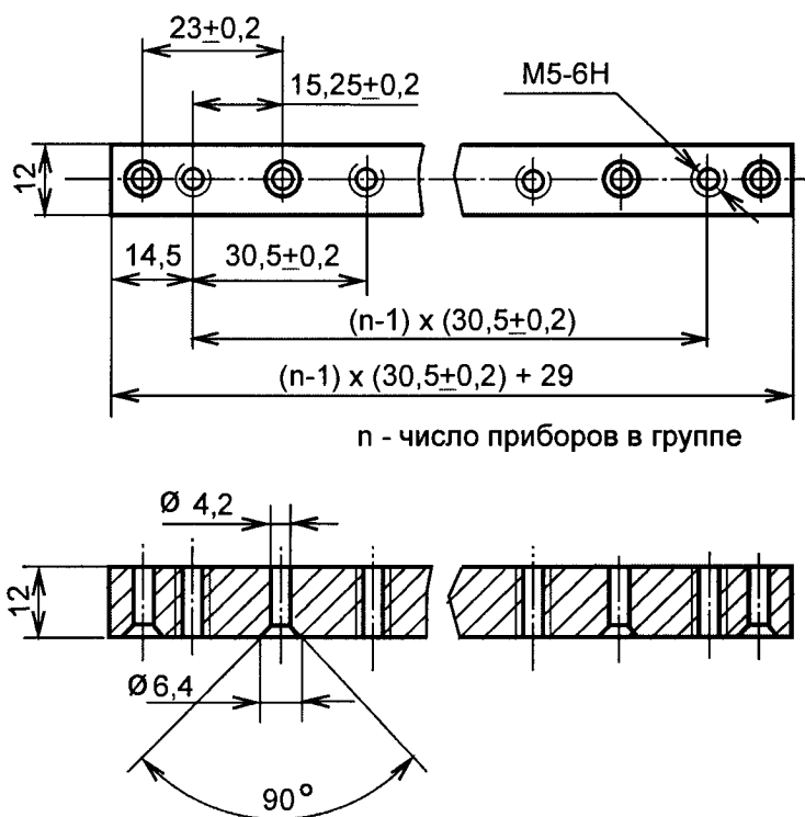
Рисунок 6 – Крепёжная планка
