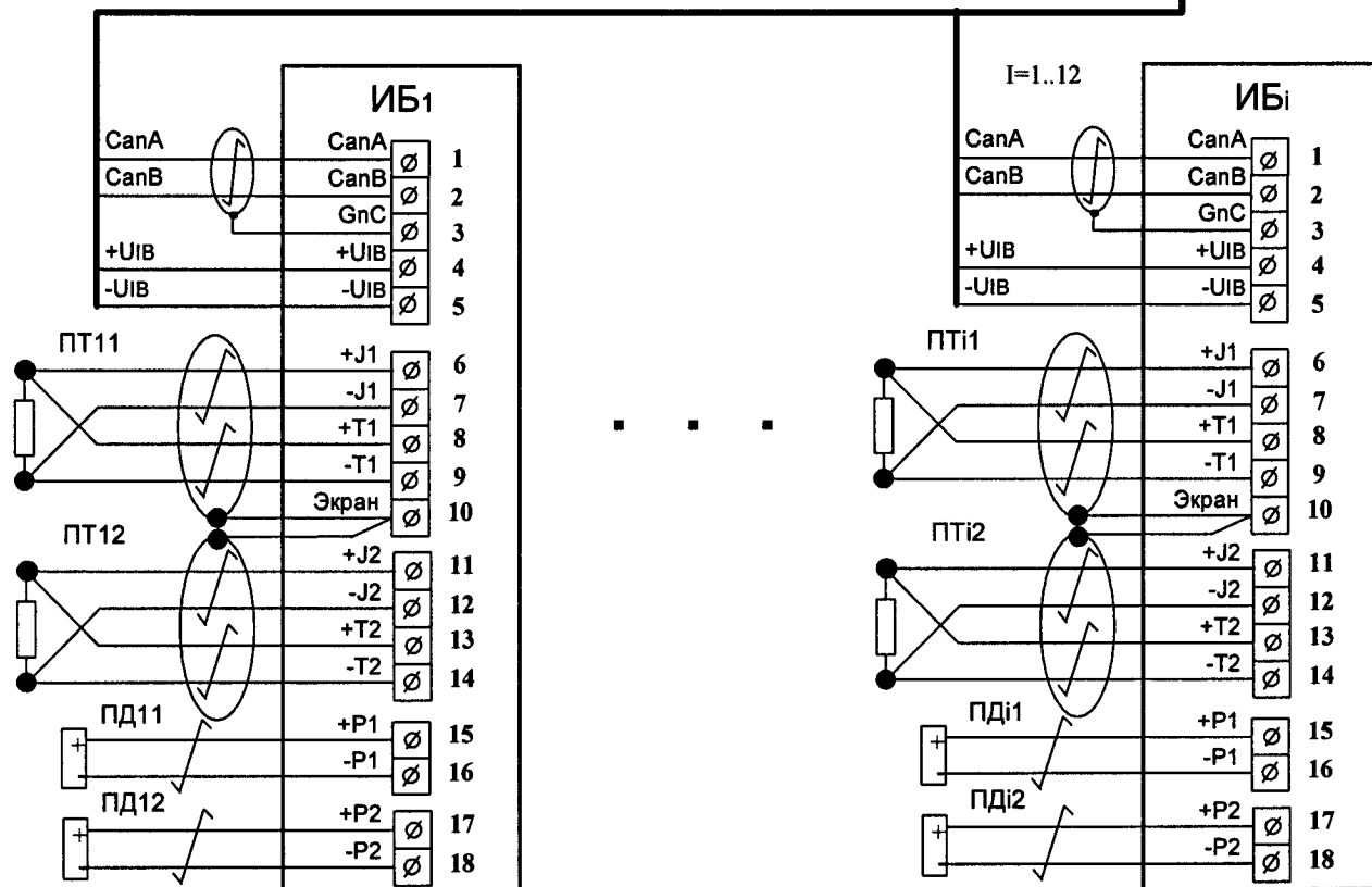
Рисунок 5.6. Электромонтажная схема многопоточного теплосчетчика с ИБ имеющим цифровые выходы.
