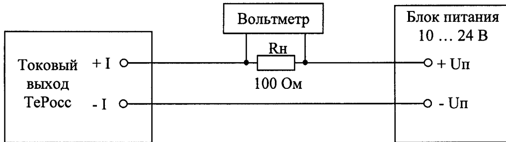
Рис. П1а. Электрическая схема подключения измерительных приборов при поверке токового выхода теплосчетчика
