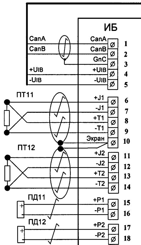
Рисунок 5.5. Электромонтажная схема однопоточного теплосчетчика с ИБ имеющим цифровой выход.
