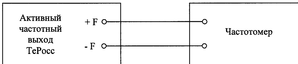
Рис. П1б. Электрическая схема подключения измерительных приборов при поверке частотного выхода теплосчетчика.
