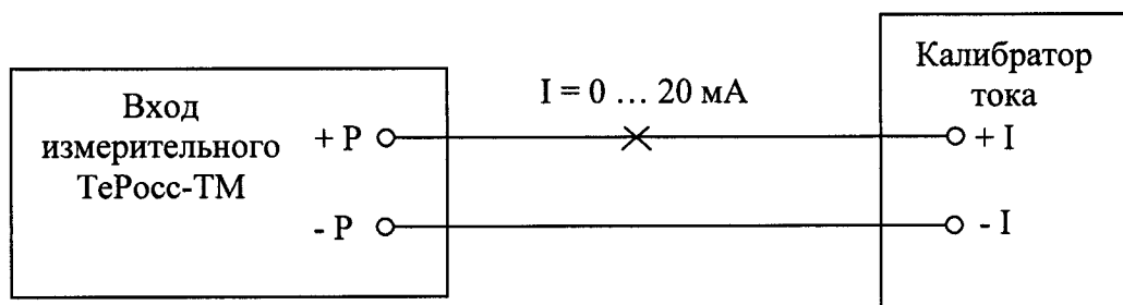
Рис. П1г. Электрическая схема подключения измерительных приборов при поверке измерительного канала давления теплосчетчика.
