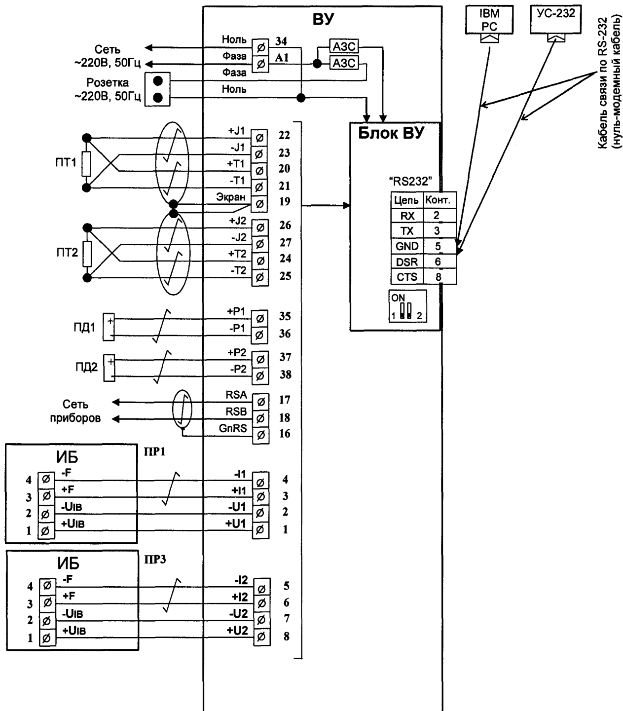
Рисунок 5.3. Электромонтажная схема двухпоточного теплосчетчика с ИБ имеющим импульсные выходы.
