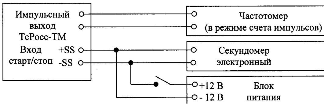
Рис. П1в. Электрическая схема подключения измерительных приборов при опробовании импульсного выхода теплосчетчика.
