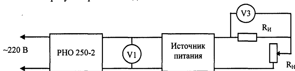
Рис. 4. Структурная схема измерения пульсации выходного тока в режиме стабилизации тока.
