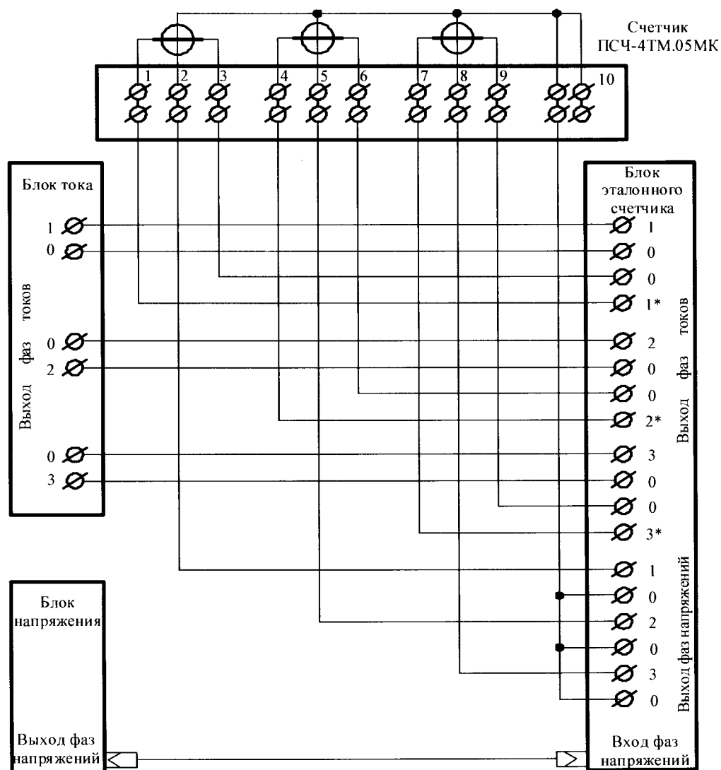
Схемы подключения счетчика к поверочной установке
