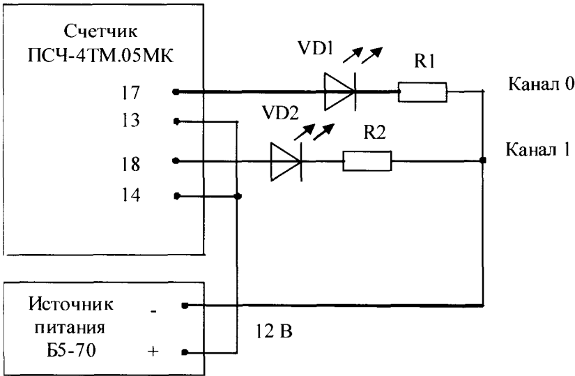
VD1, VD2 – Индикаторы единичные АЛ307БМ R1, R2- Резисторы С2-33Н-0,25-1 кОм±5 %
