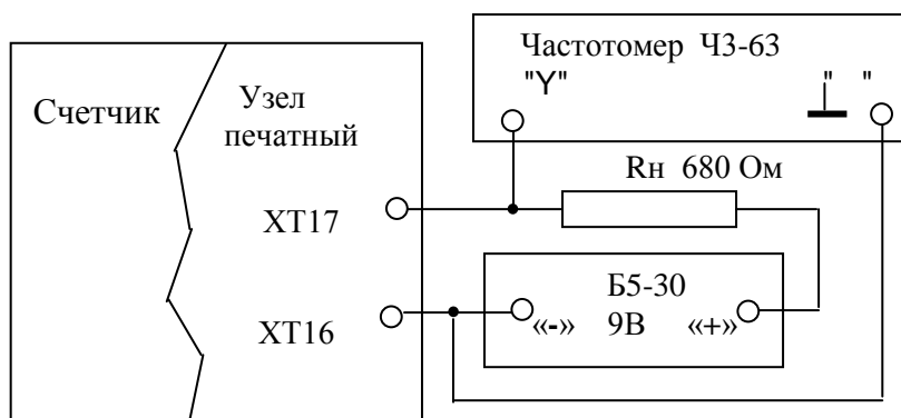
Рисунок 4 – Схема подключения оборудования для измерения точности хода часов
